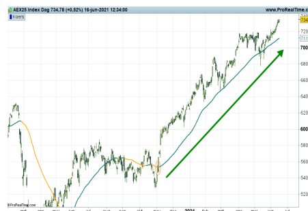
Afbeelding 2 AEX dagchart
